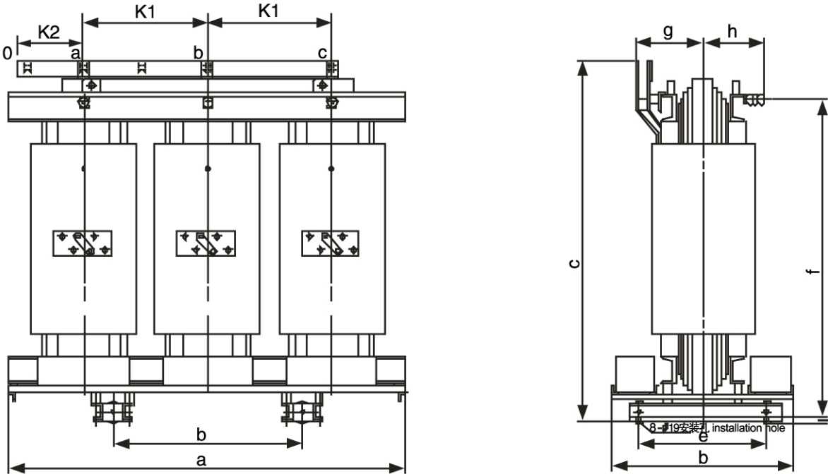
外形图二 Outline diagram 2
