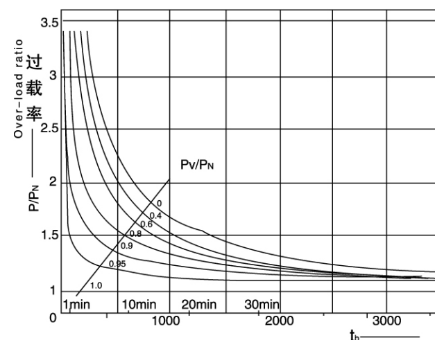
图a 环境温度 \theta_H=40^\circ\text{C} 允许过载时间 Fig.a Ambient temperature \theta_H=40^\circ\text{C} Overload time allowable
