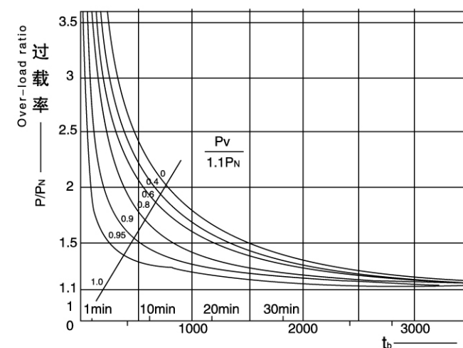
图b 环境温度 \theta_H=20^\circ\text{C} 允许过载时间 Fig.b Ambient temperature \theta_H=20^\circ\text{C} Overload time allowable
