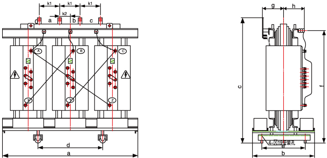
外形图三 Outline diagram 3
