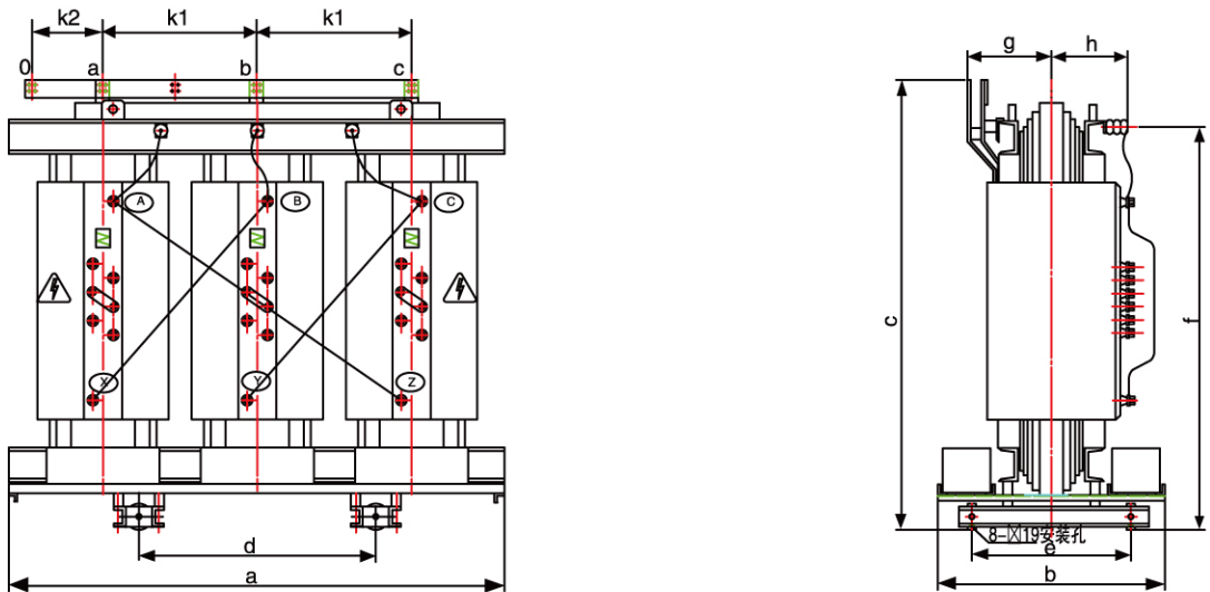
外形图四 Outline diagram 4
